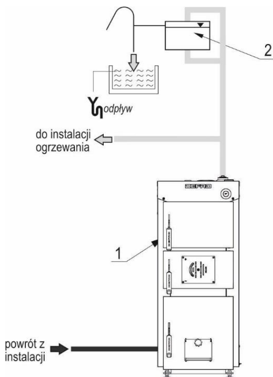
1-kocioł; 2-otwarte naczynie wzbiornicze.
