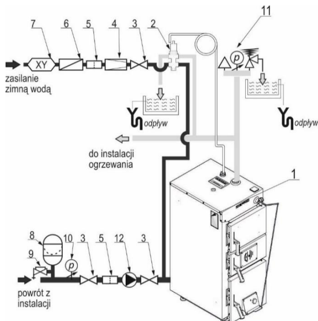
1-kocioł; 2-zabezpieczenie termiczne przed przegrzaniem /np. zawór 544/; 3-zawór kulowy; 4-reduktor ciśnienia; 5-filtr wody użytkowej; 6-zawór zwrotny; 7-zawór antyskażeniowy; 8-naczynie przeponowe; 9-zawór kołpakowy; 10-manometr; 11-armatura bezpieczeństwa; 12-pompa.
