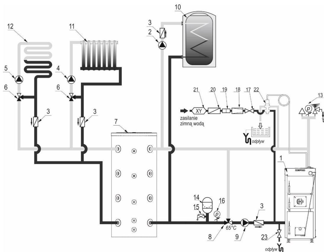
Rysunek 9. Uproszczony schemat instalacji grzewczej systemu zamkniętego.
