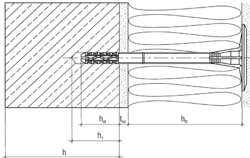
Montaż powierzchniowy
