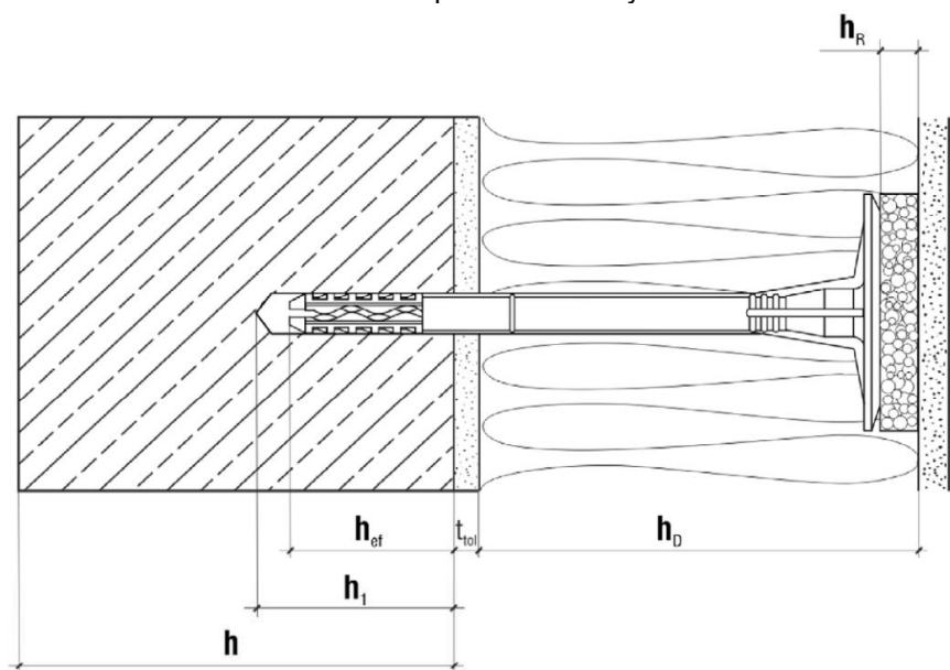
Montaż zagłębiony
